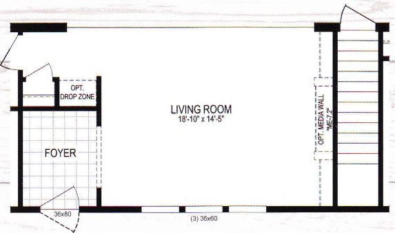
OPTIONAL BASEMENT STAIRWELL
